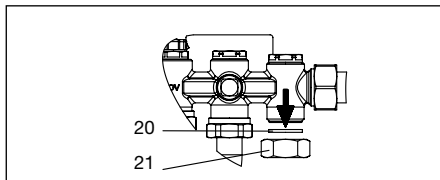
Abb. 6.1 Demontage
