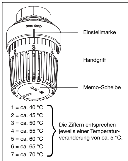
Abb. 8.3 Einstellung Trinkwassertemperatur
