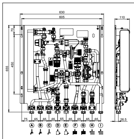
Fig. 4.2 Dimensioni con circuito alte temperature
