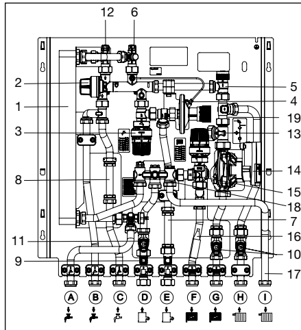
Abb. 5.1 Aufbau mit Hochtemperaturkreis
