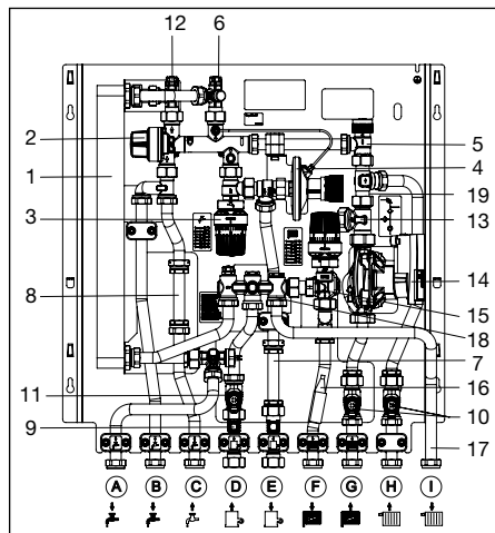
Fig. 5.1 Conception avec circuit à haute température
