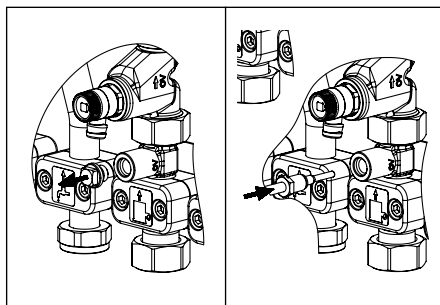
Fig. 6.3 Montage du bouchon
