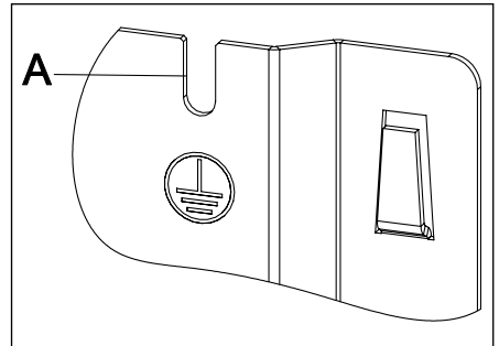
Abb. 7.1 Schutzpotentialausgleich/Erdung
