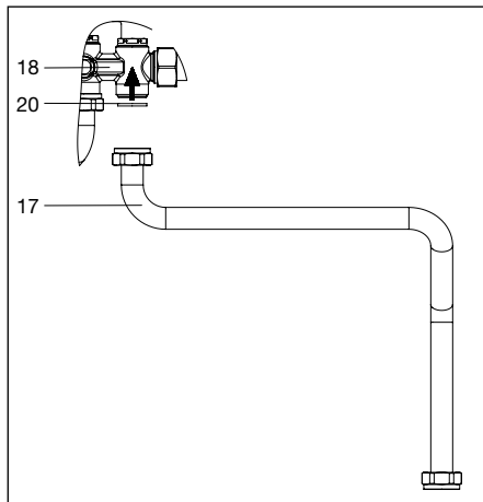
Fig. 6.2 Assemblaggio / Rimozione
