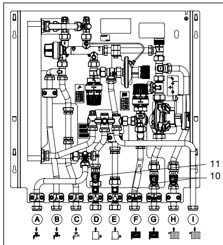
Abb. 8.1 Einbauposition Schmutzfänger
