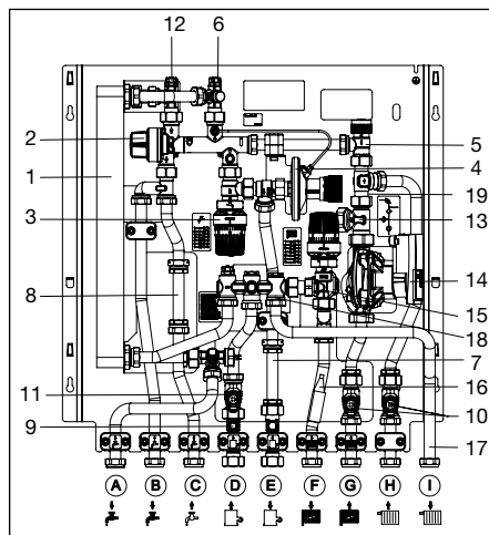
Fig. 5.1 Versione con circuito alte temperature
