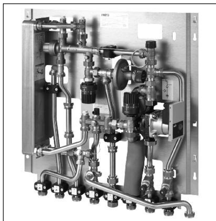
Fig. 1.1 Station d'appartement «Regudis W-HTF» avec circuit à haute température
