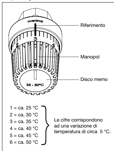
Fig. 8.4 Impostazione temperatura mandata circuito di riscaldamento
