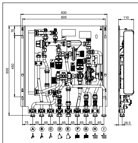
Fig. 4.2 Encombrements avec circuit à haute température
