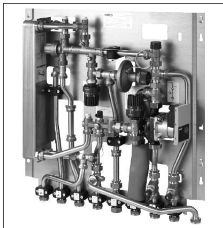
Abb. 1.1 „Regudis W-HTF“ Wohnungsstation mit Hochtemperaturkreis
