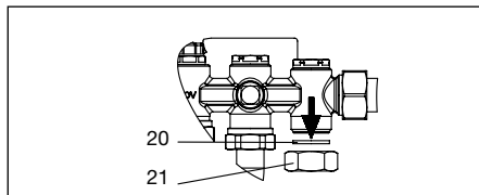
Fig. 6.1 Démontage
