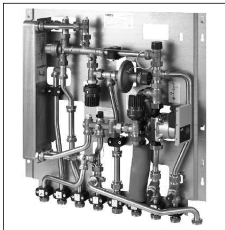
Fig. 1.1 Modulo satellite „Regudis W-HTF“ con circuito alte temperature
