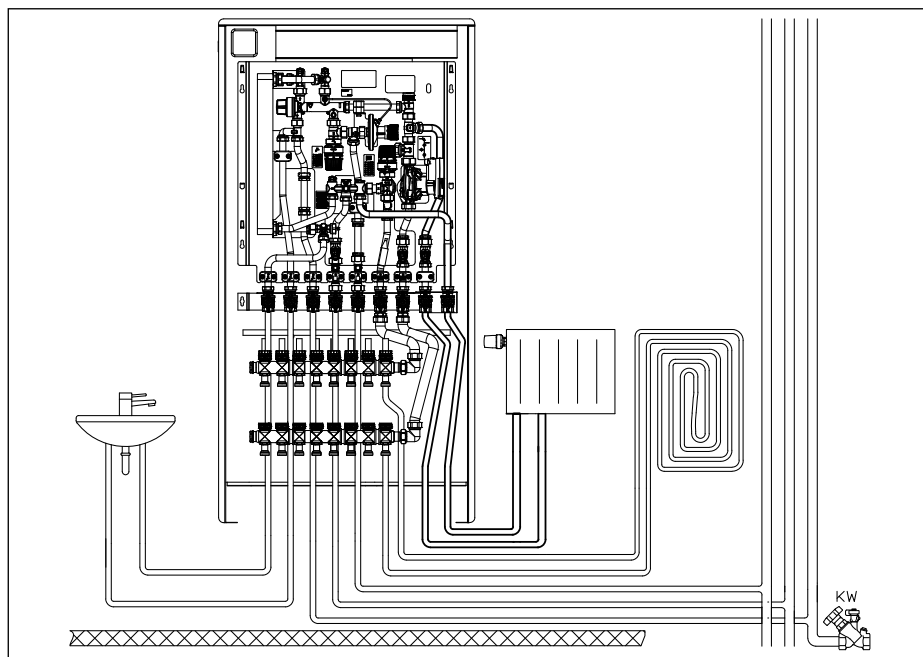
Fig. 8.5 Exemple d'installation
