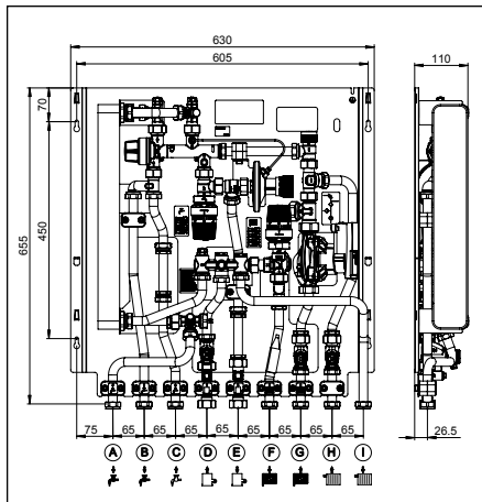
Abb. 4.2 Abmessungen mit Hochtemperaturkreis
