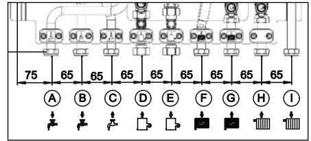
Abb. 4.3 Anschlussmaße
