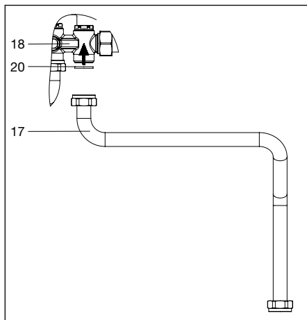
Abb. 6.2 Montage
