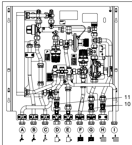
Fig. 8.1 Posizione di montaggio filtro
