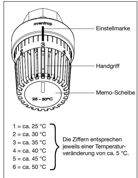
Abb. 8.4 Einstellung Vorlauftemperatur Heizkreis
