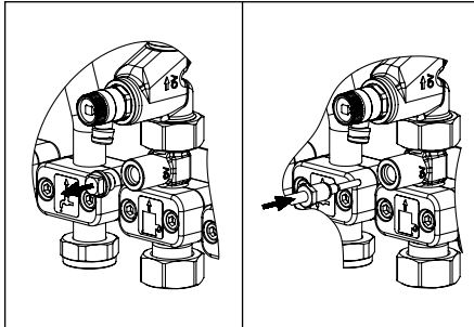
Abb. 6.4 Einbau Fühler für Wärmehähler
