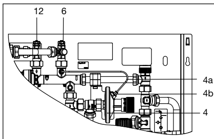
Fig. 8.2 Purge
