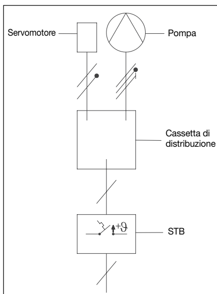
Fig. 4.1 Schema cablaggi
