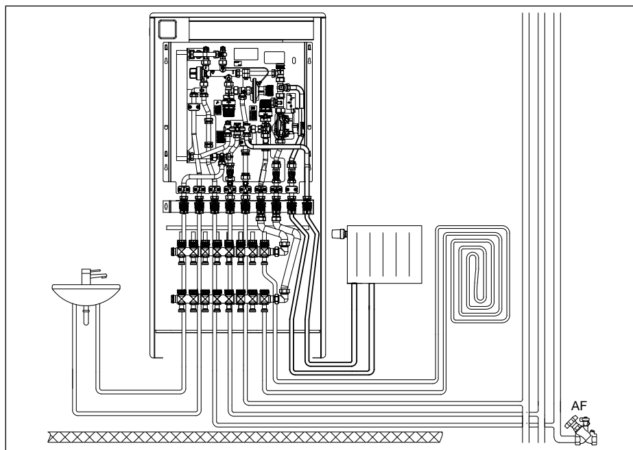
Fig. 8.5 Esempio applicativo
