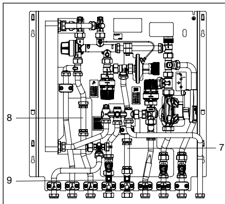
Fig. 6.3 Montage du compteur d'eau froide et du compteur de calories
