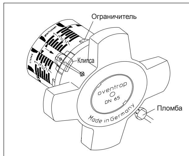
Рис. 3: блокировка и пломбировка настройки
