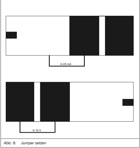
Abb. 8: Jumper setzen
