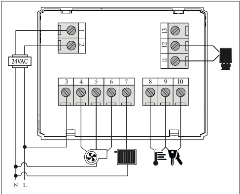
Fig. 5: Schéma de raccordement 1152064
