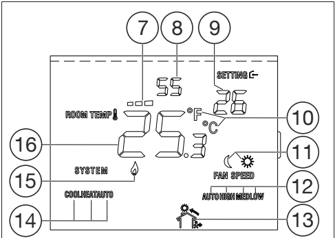
Fig. 3: Affichage digital
