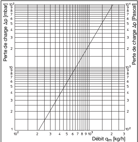
Diagramme 1: Perte de charge jeu de raccordement no. 1 pour compteurs de calories, DN20
