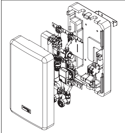
Abb. 5.1: Gesamtansicht Armaturenbaugruppe
