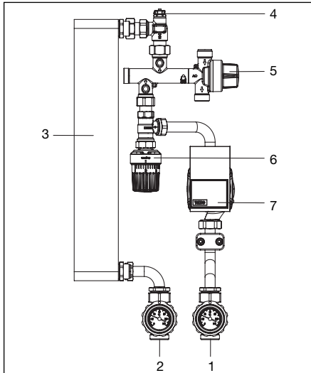
Abb. 5.2: Primärkreislauf
