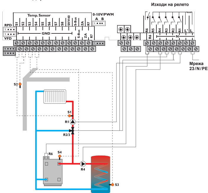
Схема 5: смесен отоплителен кръг с нагряване на битовата вода и допълнително отопление (запитване за отоплителен кръг и битовата вода)
