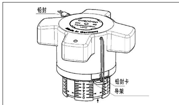
图 7.2 手轮的锁定
