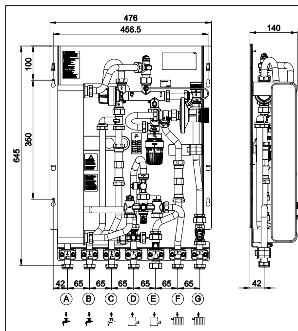
Maße
