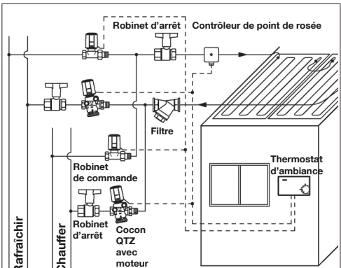
Fig. 7: Exemple de montage 1: Système à quatre tuyaux
