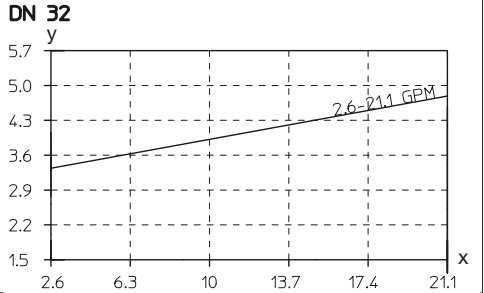
Fig. 13: Pressions différentielles min
