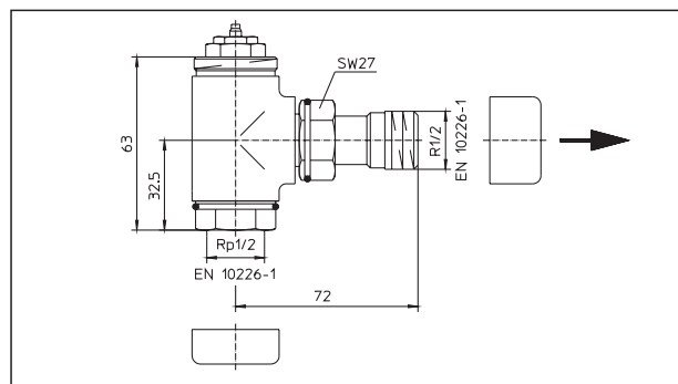
Corps de robinet équerre
