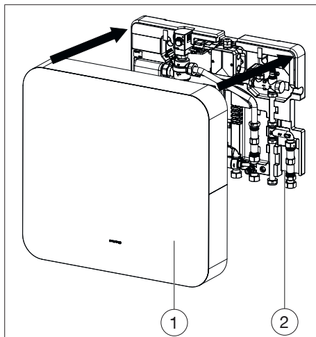
Abb. 2: Montage Wärmedämmoberschale
