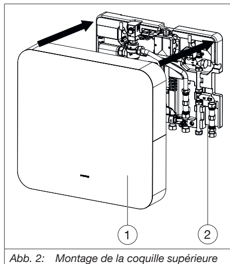
Abb. 2: Montage de la coquille supérieure
