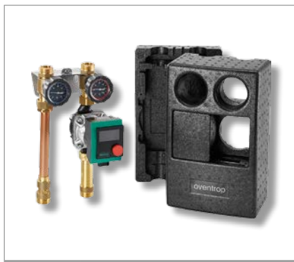
"Regumat S-130" DN 20 – circuito de calefacción de temperatura constante
