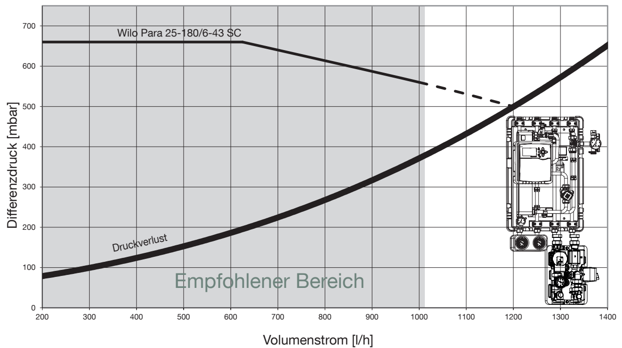
Abb. 5: Druckverlust Sekundärkreis Regudis H-MT
