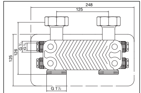
„Regumat“ Wärmeübertrager
