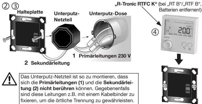
Abbildung 9: Wandmontage Halteplatte „R-Tronic“ mit Unterputznetzteil
