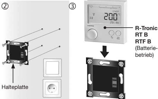
Abbildung 8: Wandmontage Halteplatte (Batteriebetrieb)
