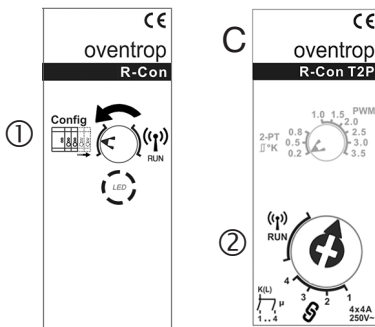
Abbildung 21: Neukonfiguration „R-Con“ nach Einbau Erweiterungsmodul
