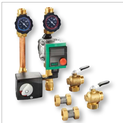
Anbaugruppe Heizkreis
