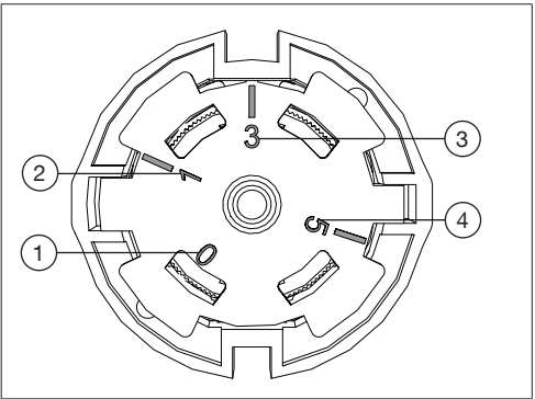
Abb. 4: Einstellmöglichkeiten Fühlereinheit
