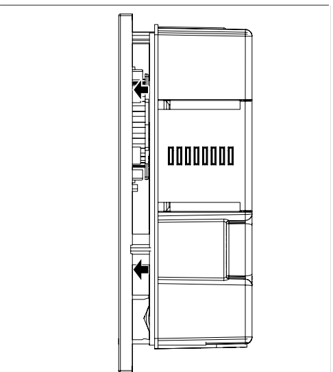
Abb. 11: Abdeckung herausgeschoben
