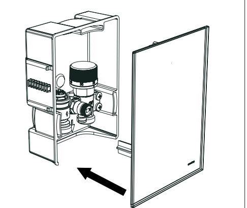
Abb. 10: Abdeckung aufsetzen
