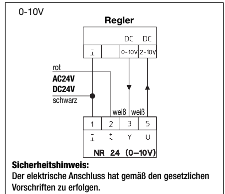
Anschluss-Schema
