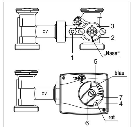
Montage 3-Wege-Mischhahn
