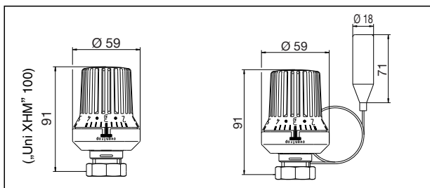
„Uni XH”, „Uni XHT” „Uni XHM” termosztátok
