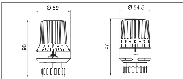
„Uni XD” termosztát
