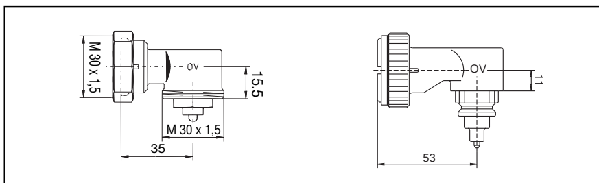
Sarokadapter, termékszám 101 14 50
