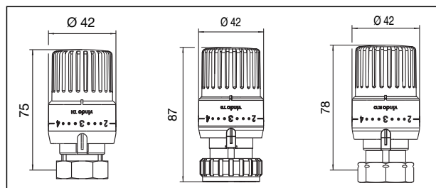
„vindo TH” termosztát
