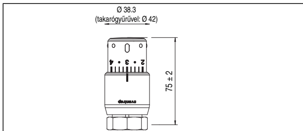
„Uni SH” termosztát
