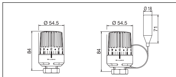
„Uni LH” termosztát
