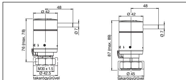
„pinox H” termosztát
