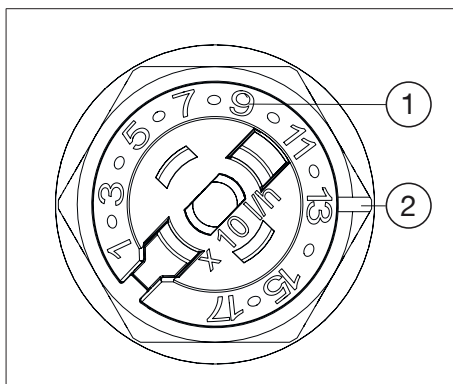
Abb. 5: Einstellung Ventileinsatz „QM“
