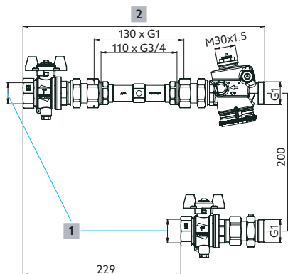
Abb. 4: Abmessungen Durchgangsausführung
