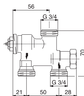
Вентиль „ТКМ“ (для однотрубных/двухтрубных систем)
