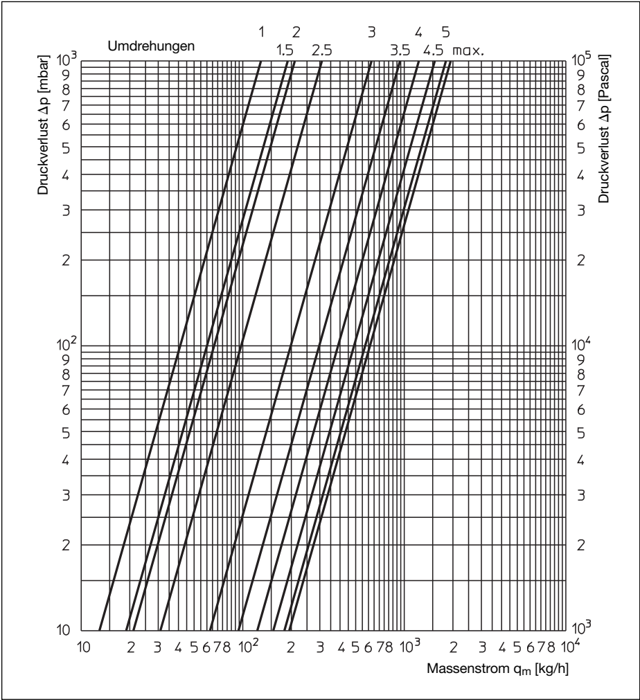
Diagramm 1: Druckverlustdiagramm Reguliereinatz bei geöffnerten Ventil
