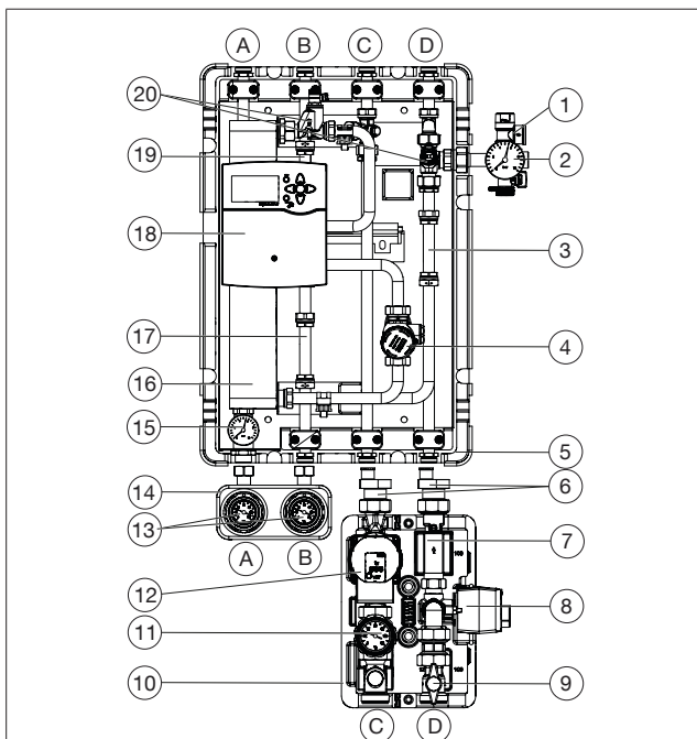
Fig. 2: Configuration Regudis H-MT
