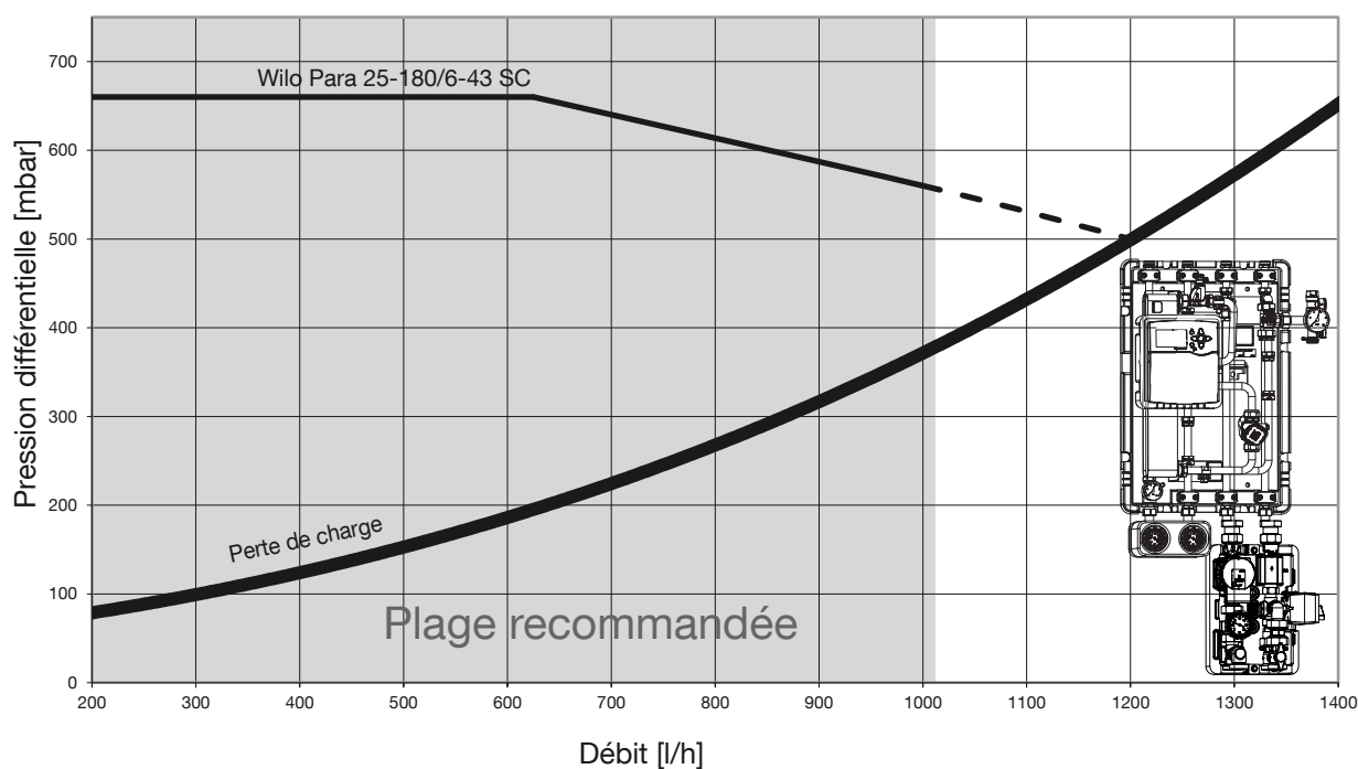
Fig. 5: Perte de charge circuit secondaire Regudis H-MT
