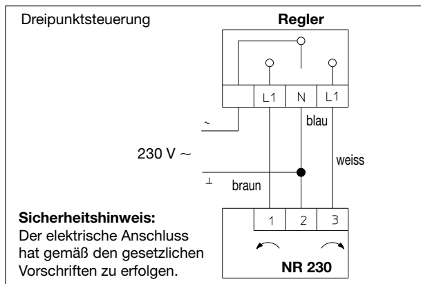
Anschluss-Schema
