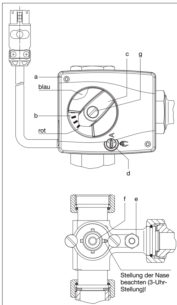
Montage Stellmotor
