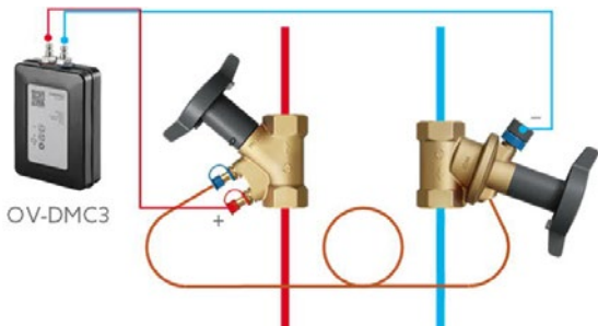
图 9： 连接图 OV-DMC3
