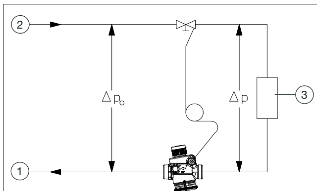
Fig. 4: Exemplu de instalare
