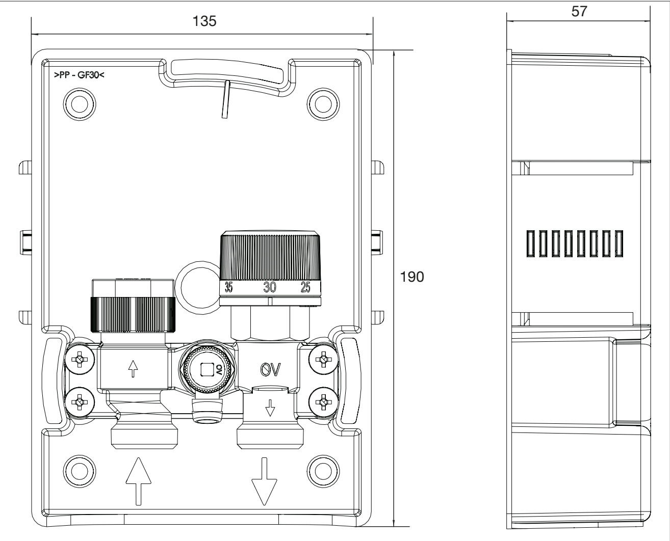
Fig. 2: Dimensiuni „Unibox TQ-RTL vario“ în mm (vedere frontală și laterală)
