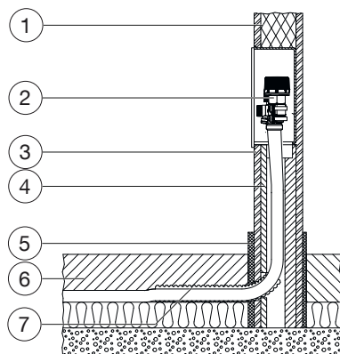
Abb. 6: Einbauquerschnitt
