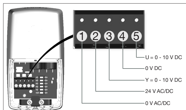
Fig. 5: Dispunerea conexiunilor
