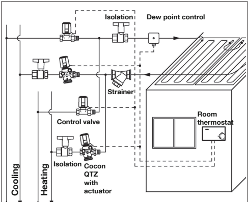
Illustr. 7: Ejemplo de instalación 2: Sistema de 4 tubos
