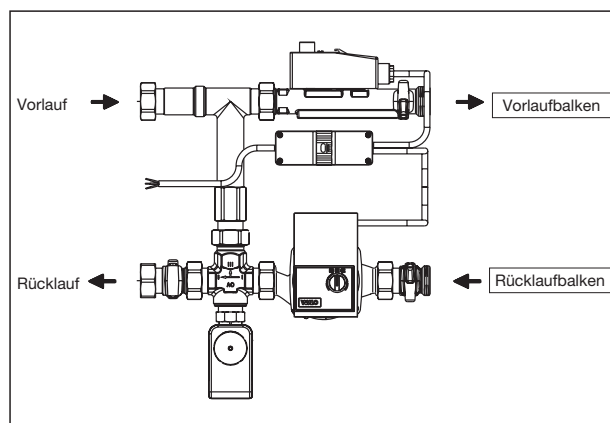
Durchflussrichtung
