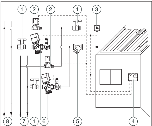
Abb. 7: Exemple de montage 2 : système à quatre tuyaux
