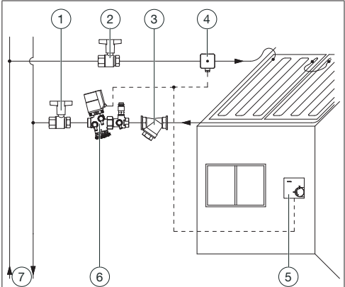
Abb. 6: Exemple de montage 1 : système à deux tuyaux
