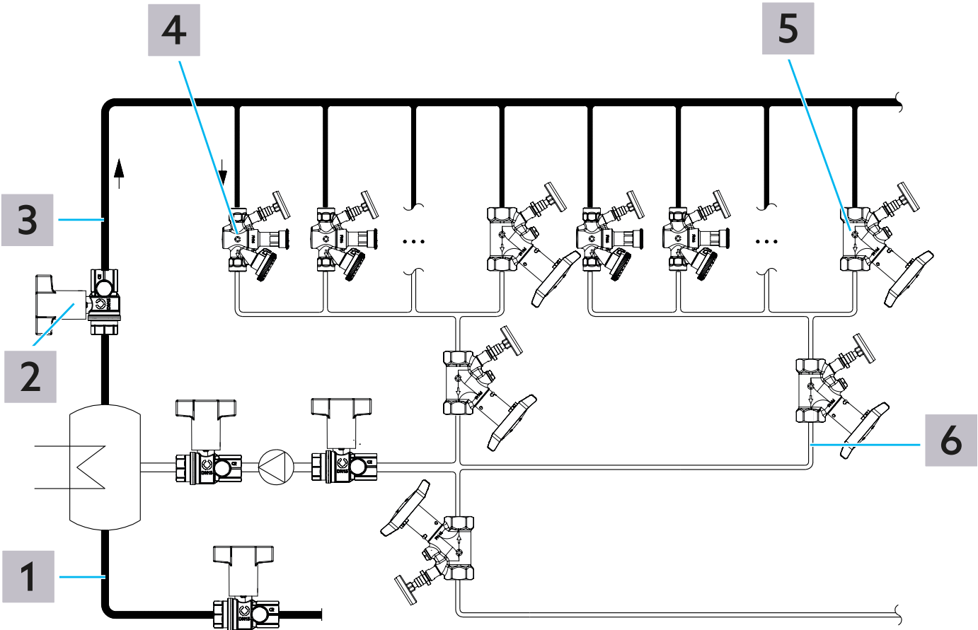
Obr. 4: Schéma zariadenia
