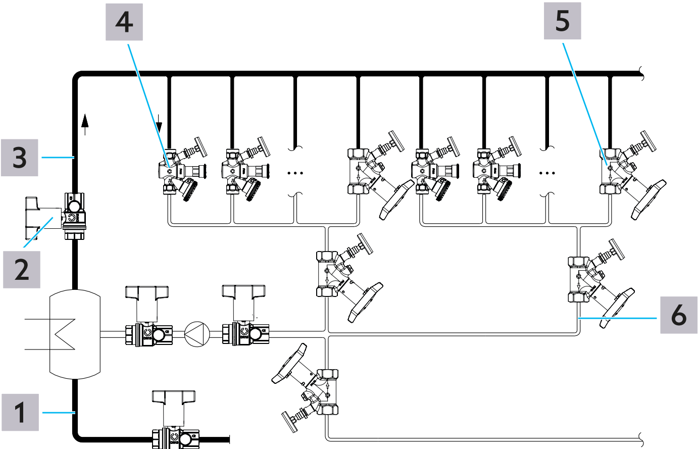
Fig. 4 - Schema dell'impianto
