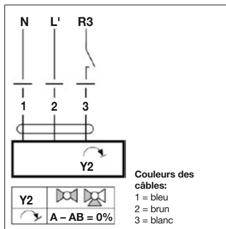
Fig. 3: Installation électrique au régulateur «Regtronic RQ»
