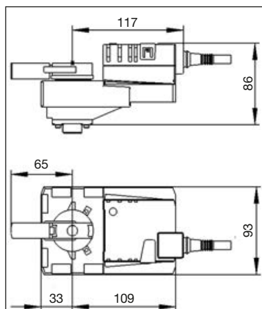
Fig. 2: Dimensions
