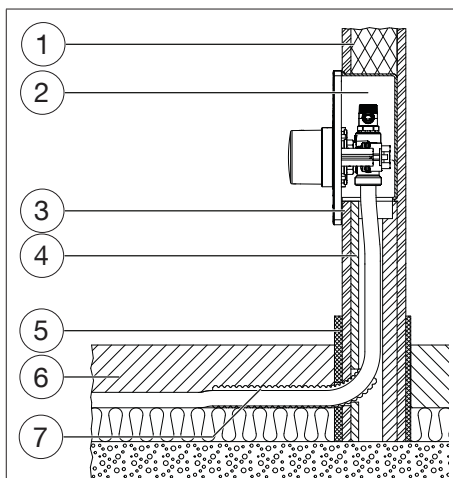
Abb. 9: Einbauquerschnitt
