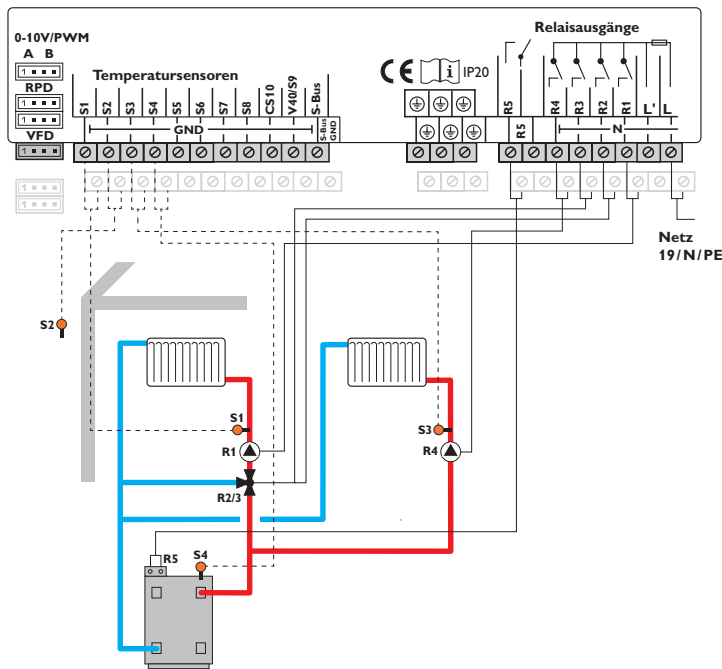
Schema 7: ein gemischter und ein ungemischter Heizkreis mit Nachheizung (Anforderung)
