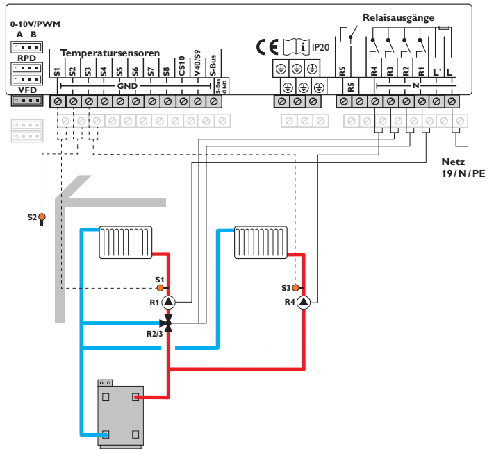
Schema 6: ein gemischter und ein ungemischter Heizkreis
