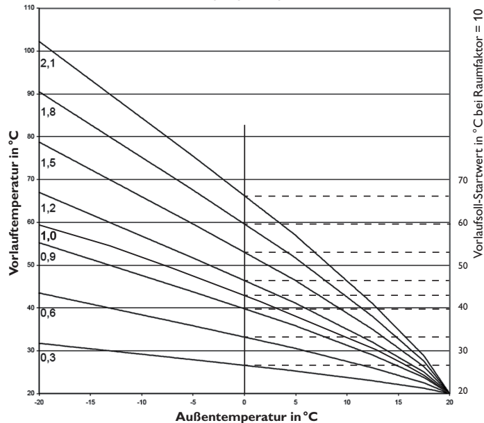
Heizkennlinien
