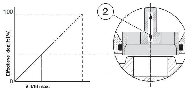
Afb. 5: Lineaire karakteristiek van regeleenheid
