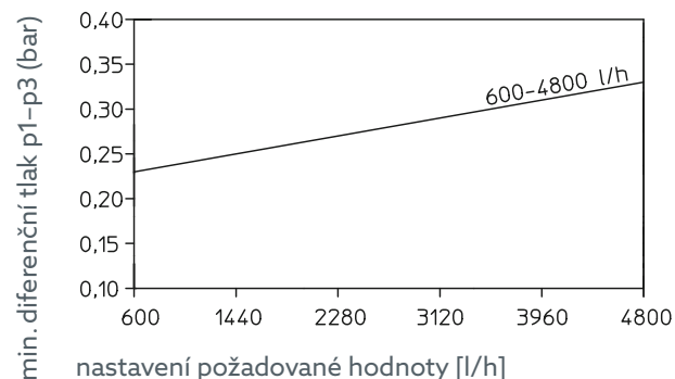
Obr. 13: Minimální diferenční tlaky
