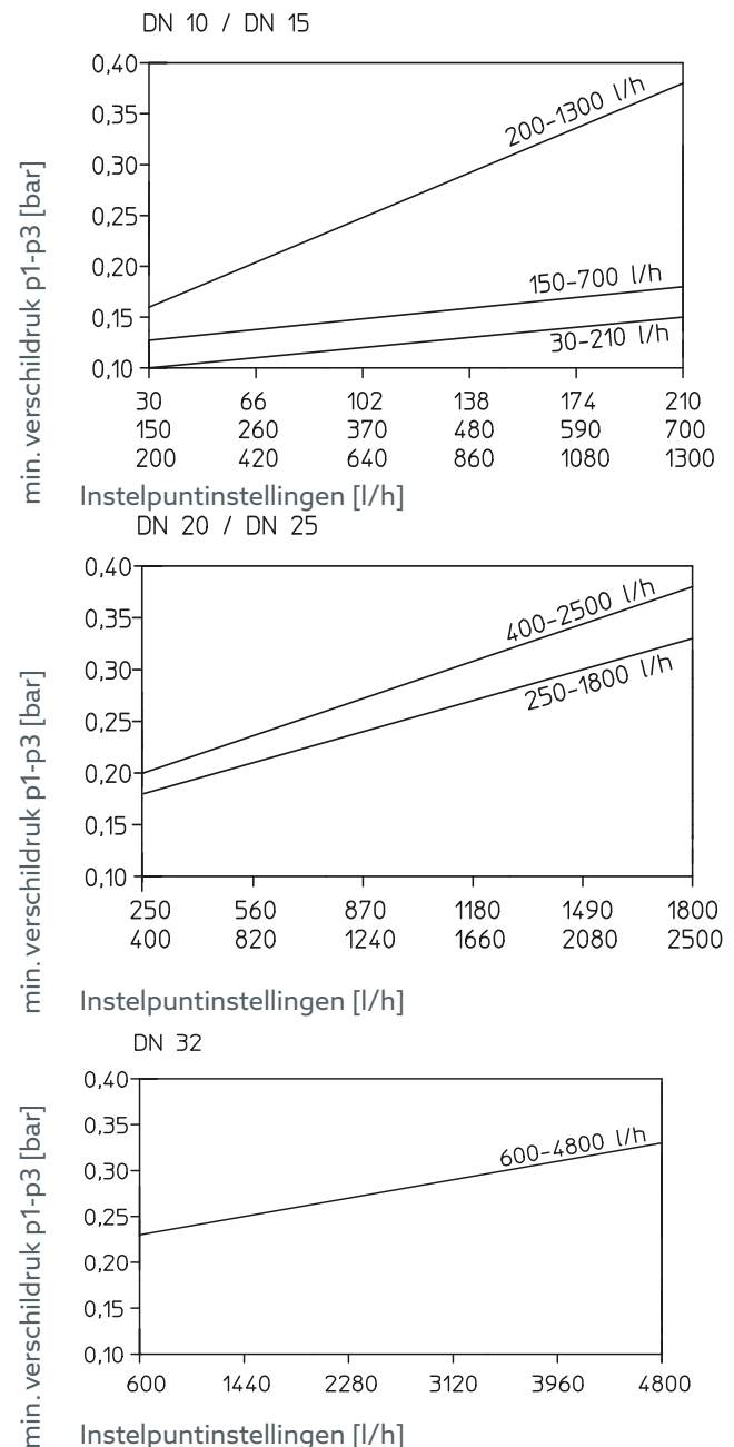
Afb. 13: Minimale verschildrukken
