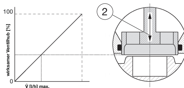
Abb. 5: Lineare Kennlinie der Reguliereinheit
