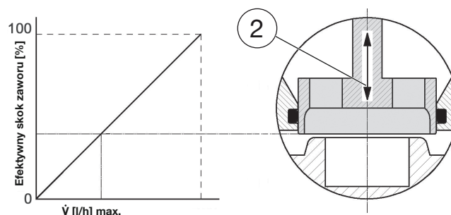
Ryc. 5: Liniowa charakterystyka zespołu regulacyjnego
