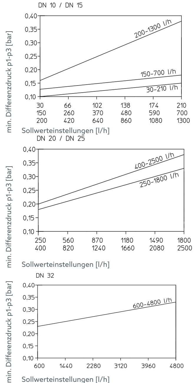
Abb. 13: Mindest-Differenzdrücke
