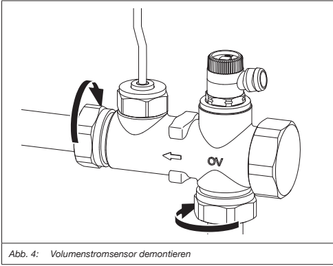
Abb. 4: Volumenstromsensor demontieren
