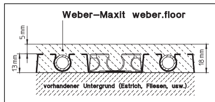
Abb. 8.3 Weber-Maxit weber.floor (Mindestüberdeckung 5 mm, Gesamtaufbauhöhe 18 mm)
