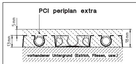
Abb. 8.2 PCI periplan extra (Mindestüberdeckung 5 mm, Gesamtaufbauhöhe 18 mm)
