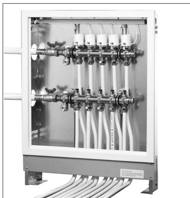
Разпределителен колектор Тип 140 40
