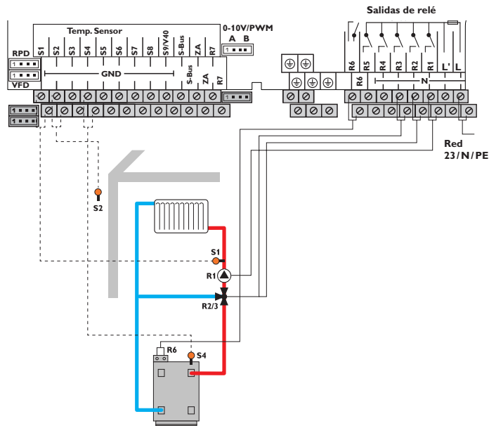
Esquema 2: un circuito de calefacción con mezcla con calentamiento auxiliar (demanda)
