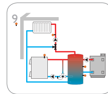
Un circuito de calefacción con mezcla, caldera de biomasa y calentamiento auxiliar
