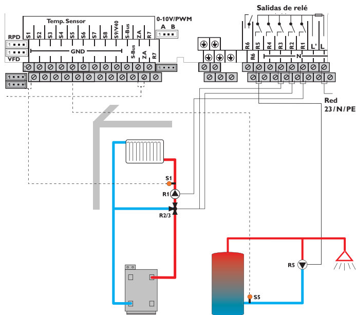
Esquema 11: un circuito de calefacción con mezcla, sonda central de temperatura exterior y circulación (secundario 2... 20)
