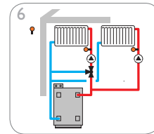
Un circuito de calefacción con mezcla y un circuito de calefacción sin mezcla
