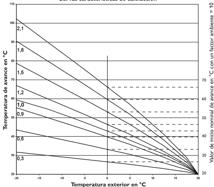
Curvas características de calefacción
