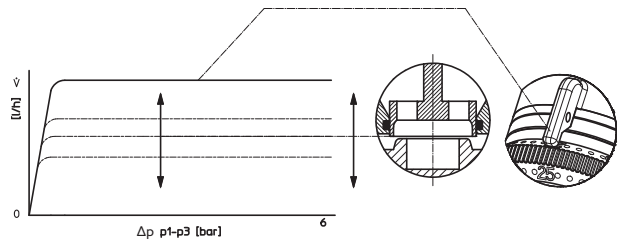
Afb. 4: Verschilddruk p1-p3 (bar)
