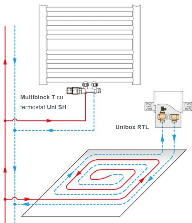
Sistem Multiblock T și Unibox RTL pentru încălzirea prin pardoseală
