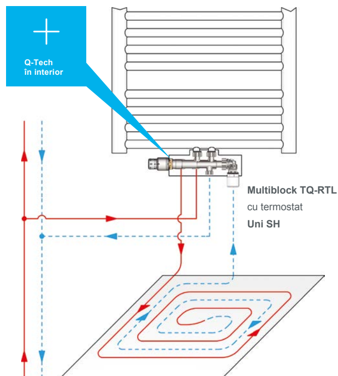
Sistem Multiblock TQ-RTL cu Q-Tech
