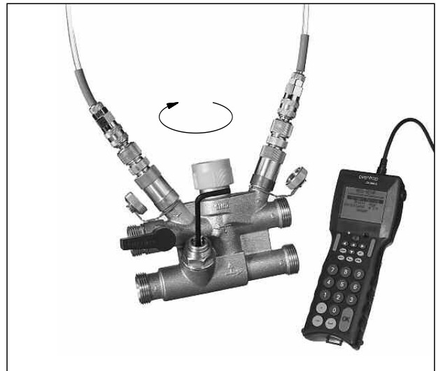
Bild 2/Illustr. 2 Voreinstellen mittels Differenzdruckmessung Presetting by differential pressure measurement Préréglage moyennant la mesure de la pression différentielle
