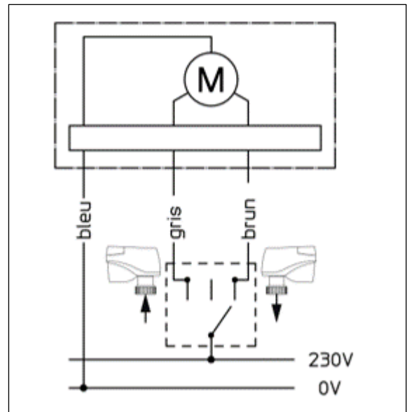
Schéma électrique, commande trois points
