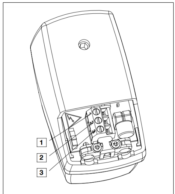
Schéma électrique, commande trois points
