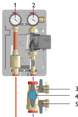
Beispiel: Solarstation mit Befüll- und Spüleinrichtung
