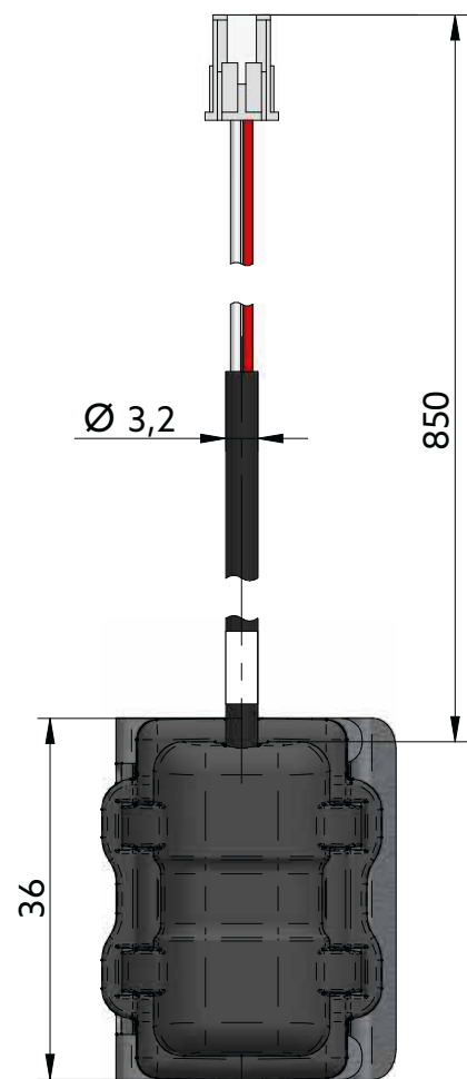
Fig. 2: Dimensions
