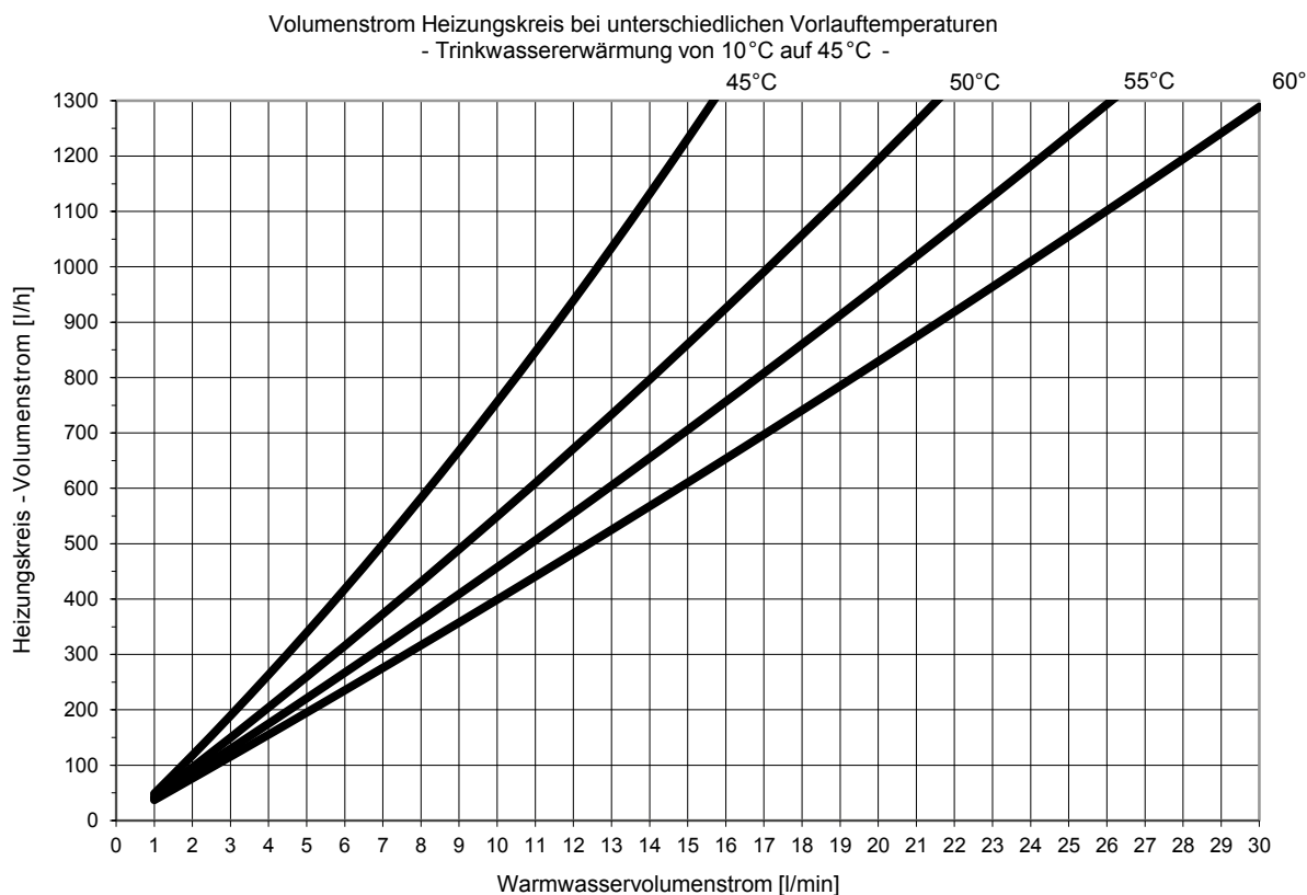
Abb. 40: Leistungsbereich 2, Trinkwassererwärmung auf 45 °C
