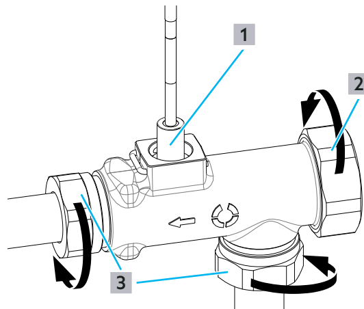
Abb. 26: Volumenstromsensor einbauen
