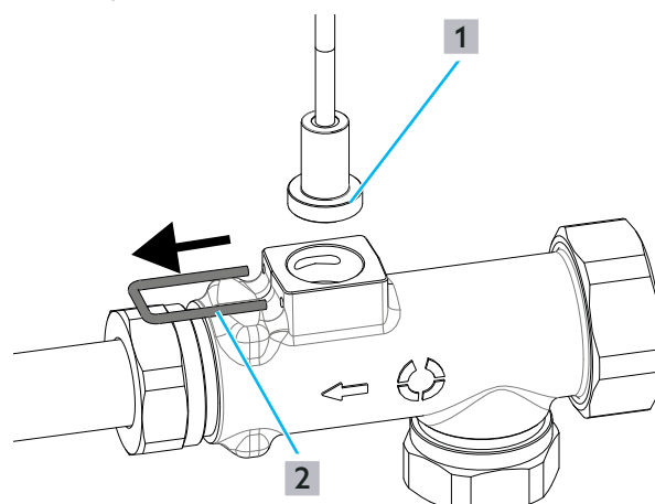
Abb. 23: Sicherungsklammer lösen
