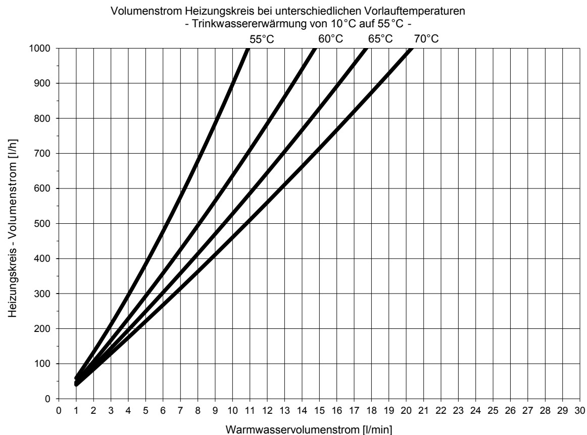
Abb. 36: Leistungsbereich 1, Trinkwassererwärmung auf 55 °C
