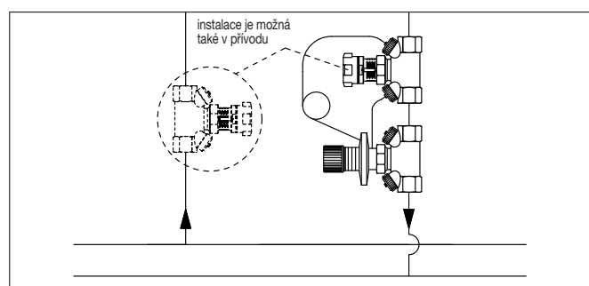
Příklad: Regulace průtoku pomocí kombinace armatur, regulátoru diferenčního tlaku „Hycococon DP“ a smyčkového regulačního ventilu „Hycococon V“
