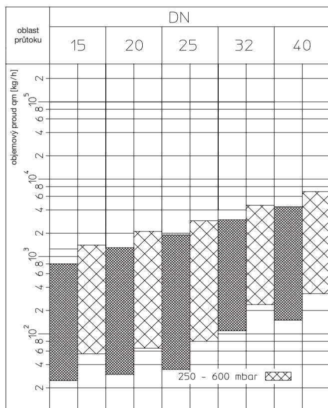
„Hycococon DP“/„Hycococon V“
