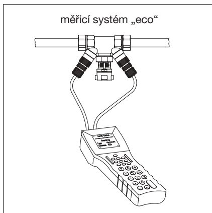
Nastavení na smyčkovém regulačním ventilu „Hycocoen V“.
