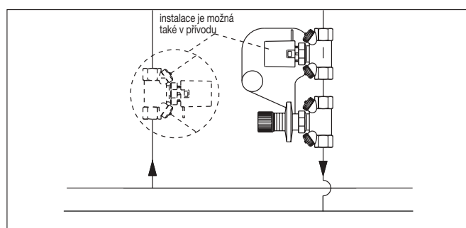
Příklad: Regulace průtoku pomocí kombinace armatur, regulátoru diferenčního tlaku „Hycococon DP“ a smyčkového ventilu „Hycococon TM“
